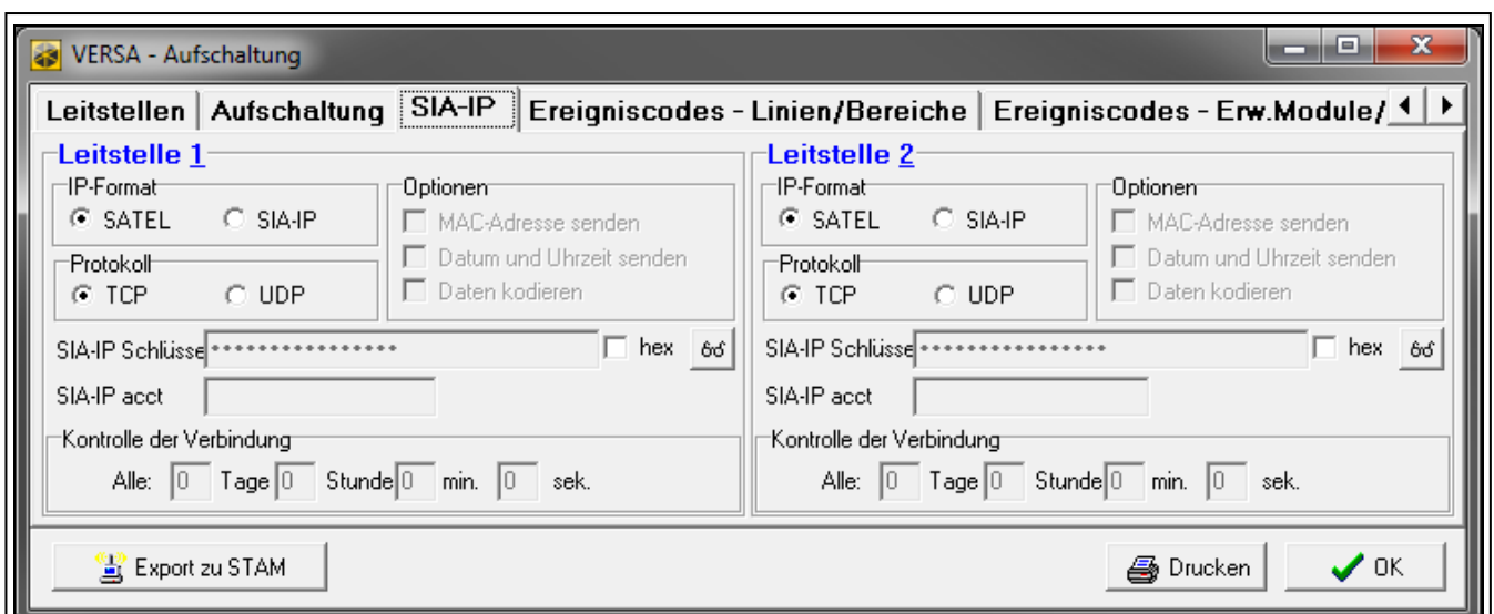
Abb. 23. Programm DLOADX: Registerkarte „SIA-IP“ im Fenster „VERSA – Aufschaltung“.
