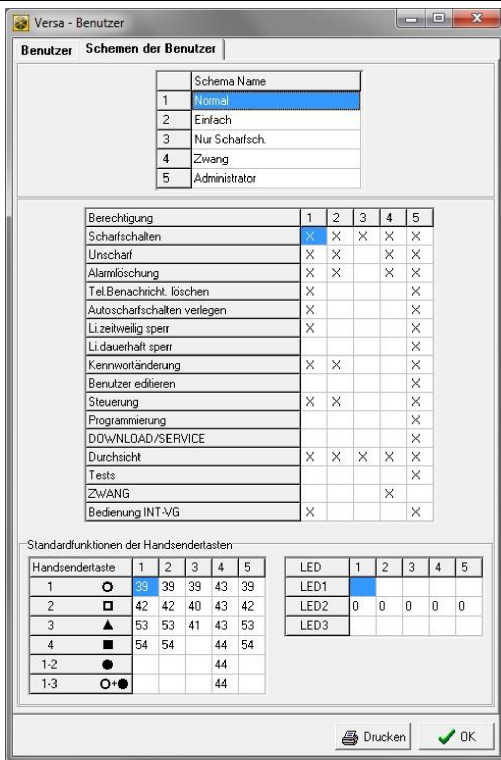
Abb. 27. Programm DLOADX: Registerkarte „Schemen der Benutzer“ im Fenster „VERSA – Benutzer“.
