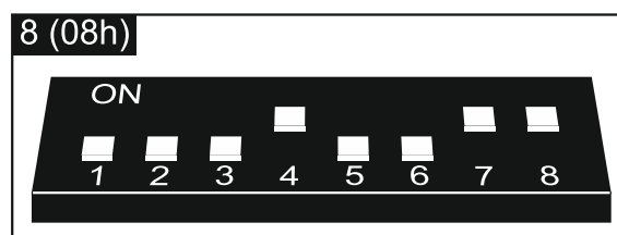
Abb. 14. Einstellung der DIP-Schalter im Modul ACU-100.
