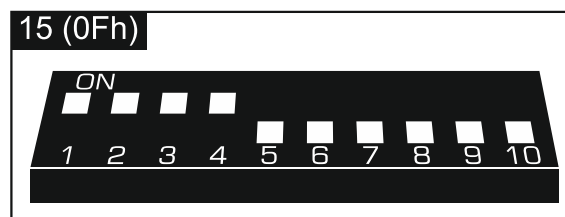
Abb. 10. Einstellung der DIP-Schalter im Modul INT-O.
