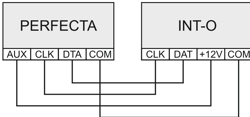
Abb. 9. Anschluss des Moduls INT-O an die Zentrale.
