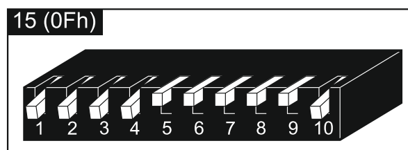
Abb. 11. Einstellung der DIP-Schalter im Modul INT-ORS.
