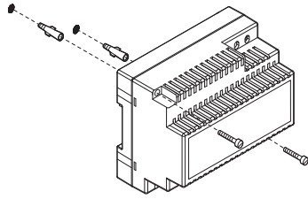
Aufputz-Installation
