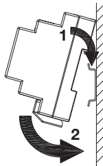
Instalación en barra DIN (6 módulos de 18 mm)
