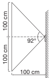
Verticaal opnameveld
