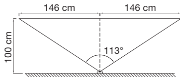
Horizontaal opnameveld
